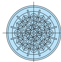
48PIN Φ38.0mm
