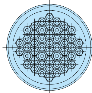
48PIN Φ38.0mm
