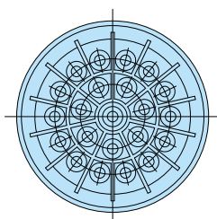
22PIN Φ28.5mm
